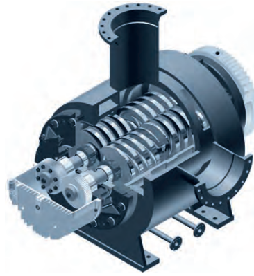
鲍诺曼双螺杆泵
